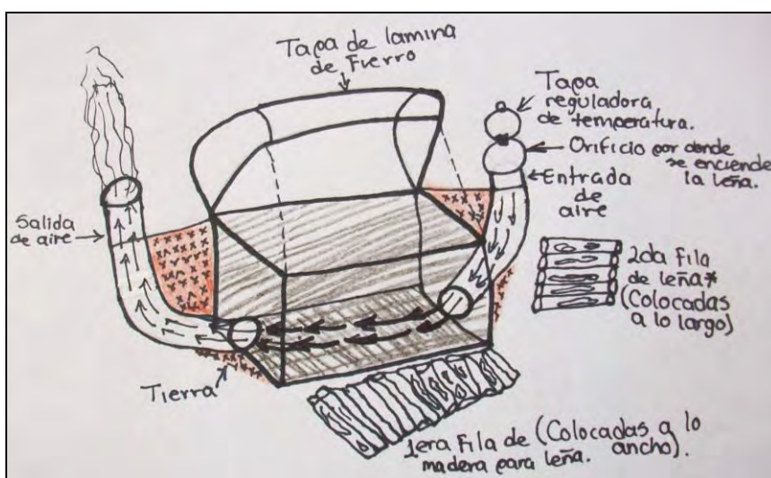
Esquema de las partes del horno para hacer carbón (Elaboración propia)
